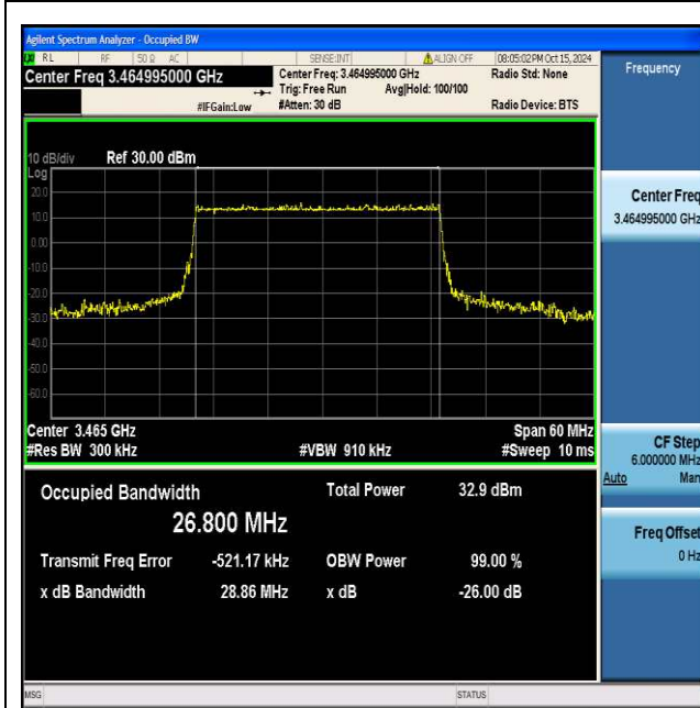
NTNV_N77-3450-3550_PC2_30_30_L_TID3_Ant1#1
