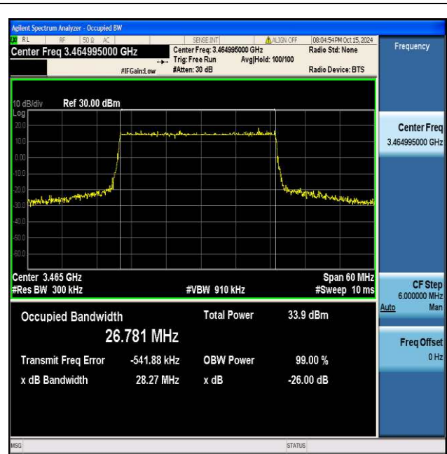
NTNV_N77-3450-3550_PC2_30_30_L_TID2_Ant1#1
