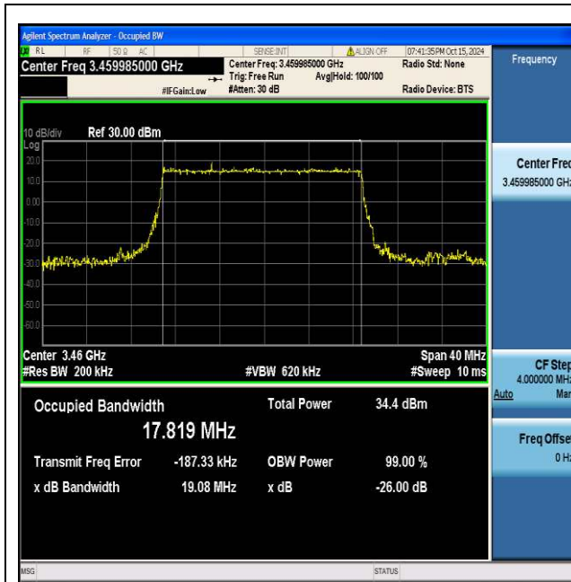
NTNV_N77-3450-3550_PC2_30_20_L_TID1_Ant1#1
