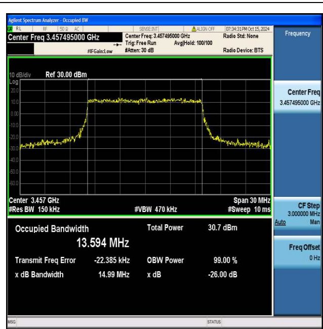
NTNV_N77-3450-3550_PC2_30_15_L_TID6_Ant1#1
