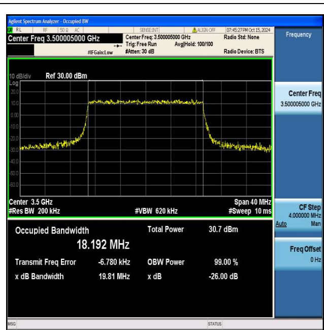
NTNV_N77-3450-3550_PC2_30_20_M_TID6_Ant1#1
