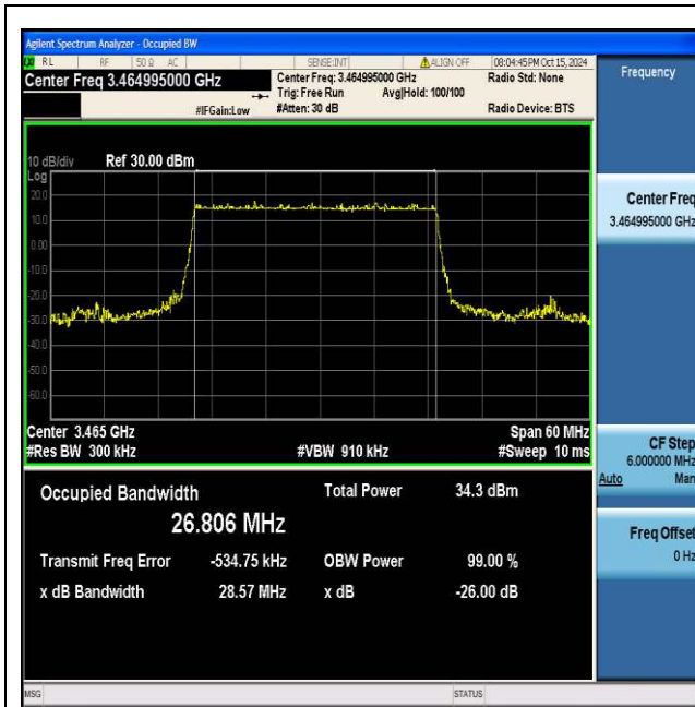
NTNV_N77-3450-3550_PC2_30_30_L_TID1_Ant1#1
