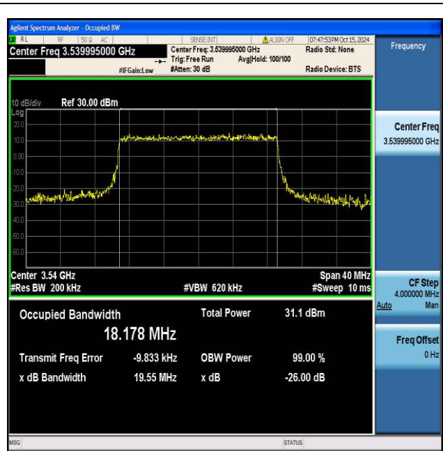
NTNV_N77-3450-3550_PC2_30_20_H_TID6_Ant1#1
