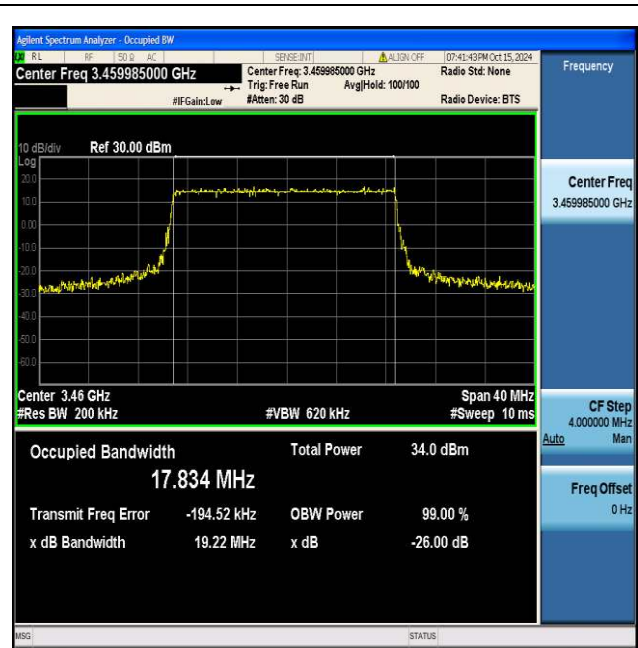
NTNV_N77-3450-3550_PC2_30_20_L_TID2_Ant1#1
