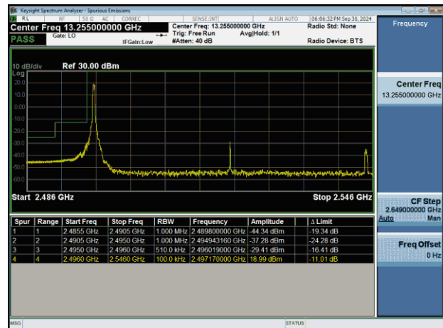
NTNV-n41-PC2-30-50-L-CP-QPSK-Edge_1RB_Left-PASS
