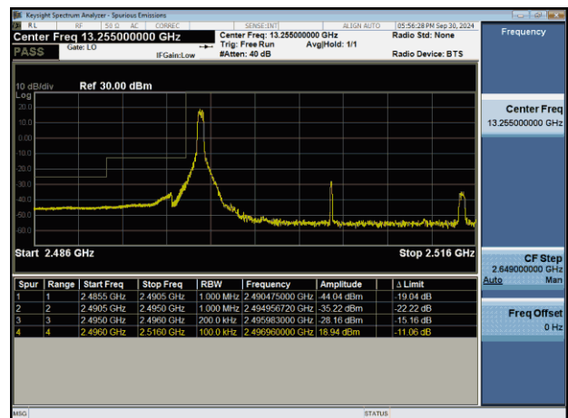
NTNV-n41-PC2-30-20-L-DFT-BPSK-Edge_1RB_Left-PASS
