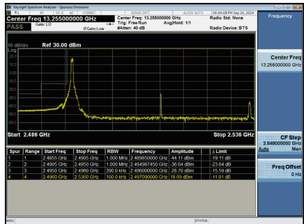
NTNV-n41-PC2-30-40-L-CP-QPSK-Edge_1RB_Left-PASS
