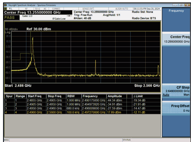
NTNV-n41-PC2-30-70-L-CP-QPSK-Edge_1RB_Left-PASS
