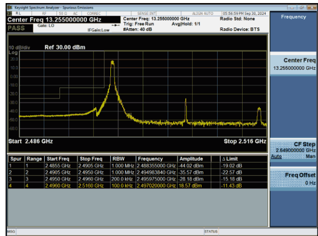
NTNV-n41-PC2-30-20-L-CP-QPSK-Edge_1RB_Left-PASS
