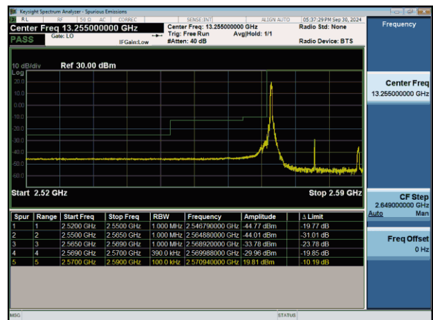
NTNV-n38-PC3-30-20-L-DFT-BPSK-Edge_1RB_Left-PASS
