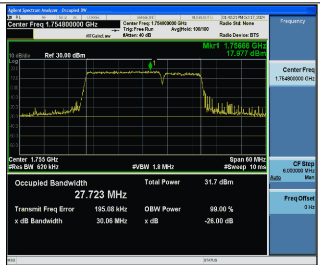
66-66-20MHz-10MHz-QPSK-QPSK-132373-132517-100RB#0-50RB#0-PASS
