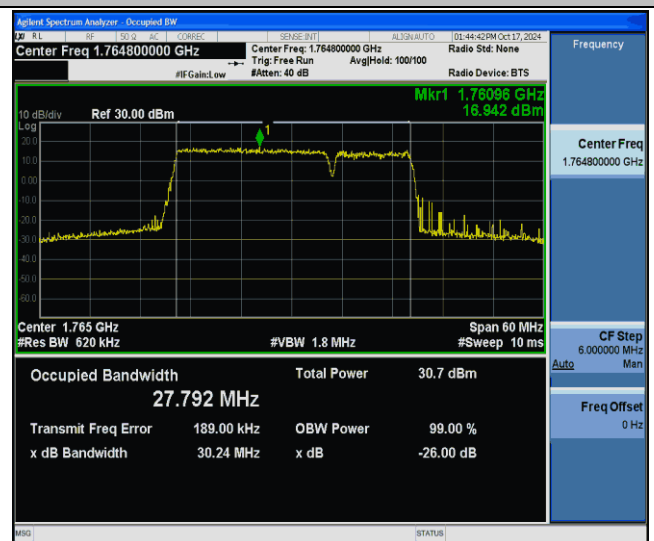
66-66-20MHz-10MHz-16QAM-16QAM-132473-132617-100RB#0-50RB#0-PASS
