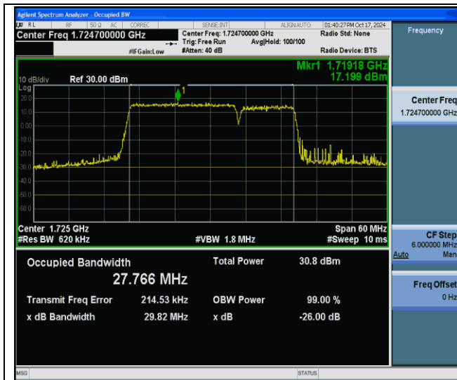
66-66-20MHz-10MHz-QPSK-QPSK-132072-132216-100RB#0-50RB#0-PASS
