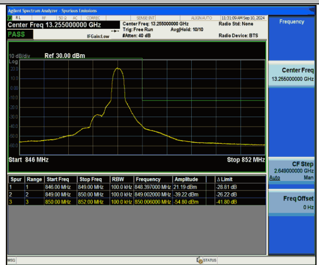
Band26(824-849)-10MHz-QPSK-26990-1RB#49-PASS
