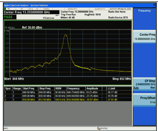
Band26(824-849)-3MHz-QPSK-27025-1RB#14-PASS
