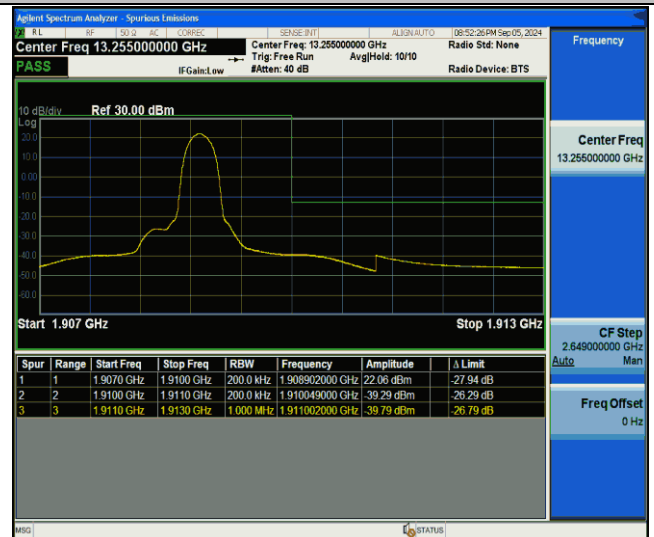
Band2-20MHz-QPSK-19100-1RB#99-PASS
