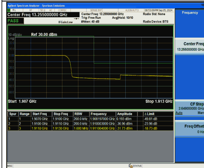
Band2-20MHz-QPSK-19100-100RB#0-PASS
