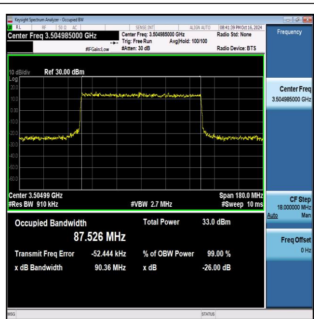
NTVN_N77-3450-3550_PC2_30_90_H_TID6_Ant1#1
