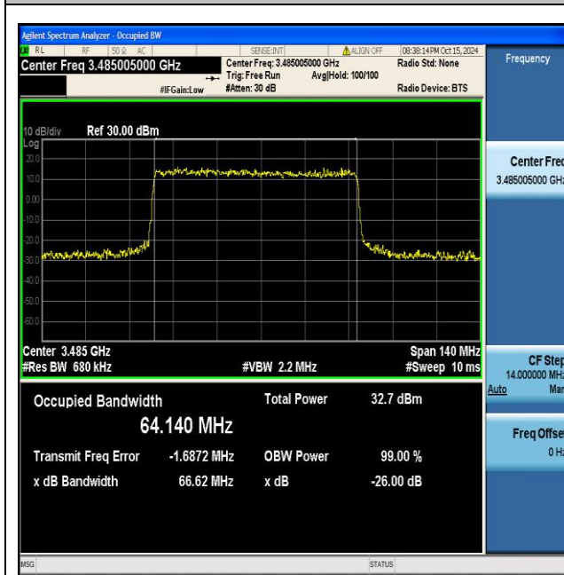
NTNV_N77-3450-3550_PC2_30_70_L_TID1_Ant1#1
