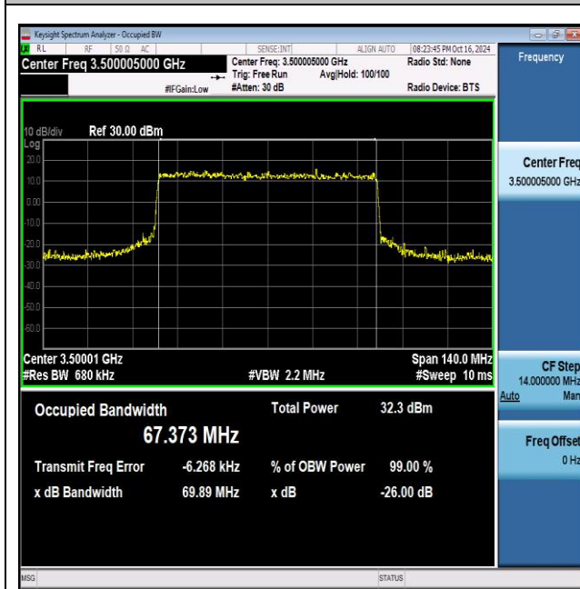
NTNV_N77-3450-3550_PC2_30_70_M_TID7_Ant1#1
