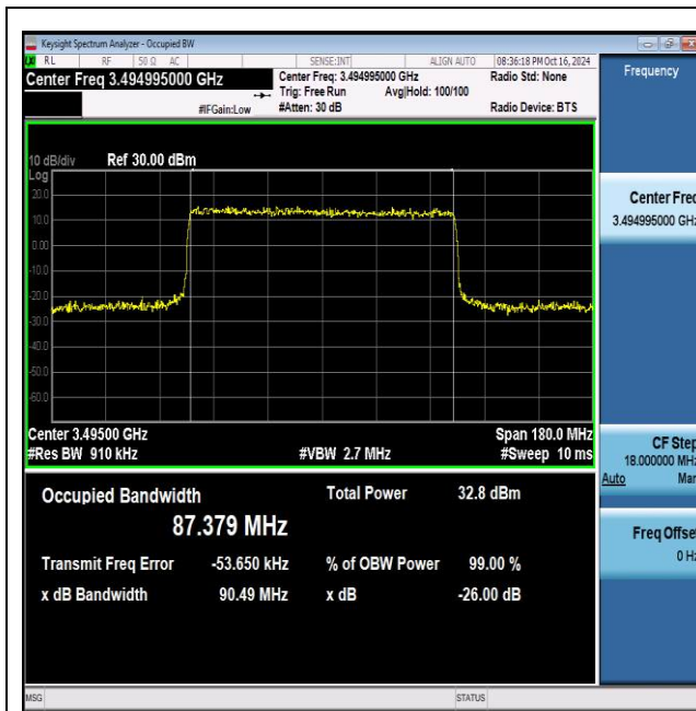
NTNV_N77-3450-3550_PC2_30_90_L_TID5_Ant1#1
