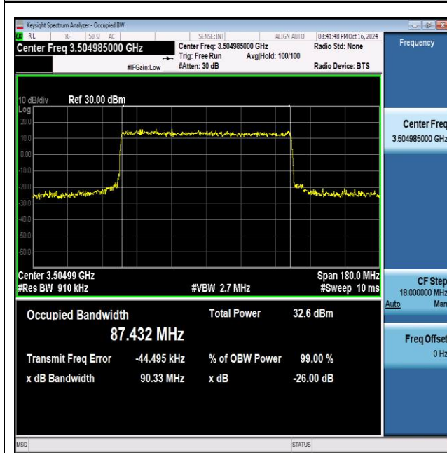
NTVN_N77-3450-3550_PC2_30_90_H_TID7_Ant1#1
