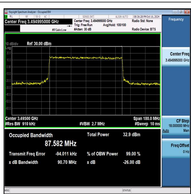
NTNV_N77-3450-3550_PC2_30_90_L_TID6_Ant1#1
