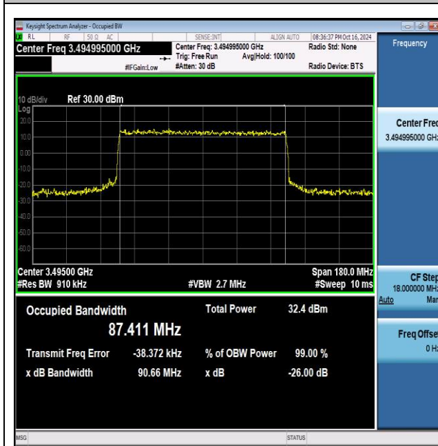
NTNV_N77-3450-3550_PC2_30_90_L_TID7_Ant1#1
