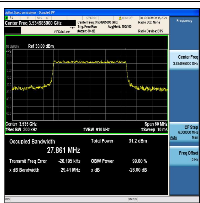
NTNV_N77-3450-3550_PC2_30_30_H_TID6_Ant1#1
