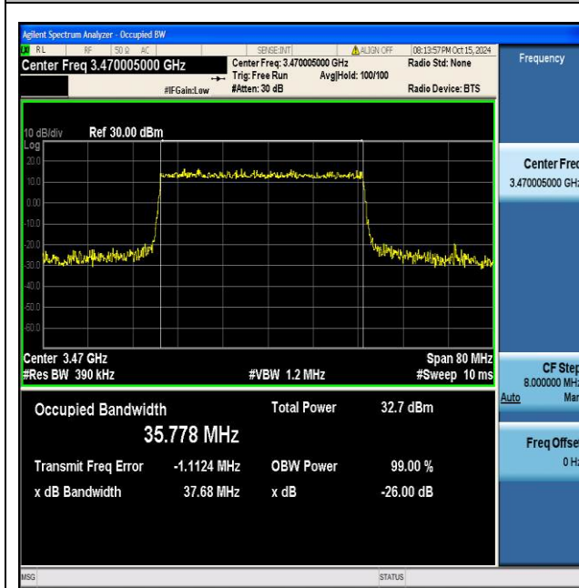
NTNV_N77-3450-3550_PC2_30_40_L_TID3_Ant1#1
