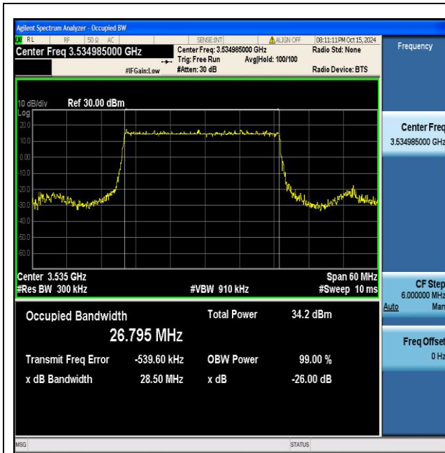
NTNV_N77-3450-3550_PC2_30_30_H_TID1_Ant1#1
