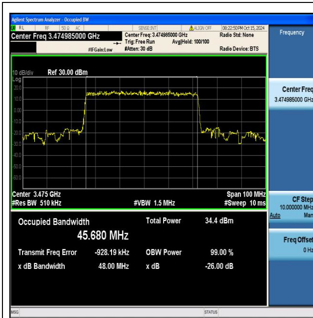
NTNV_N77-3450-3550_PC2_30_50_L_TID1_Ant1#1
