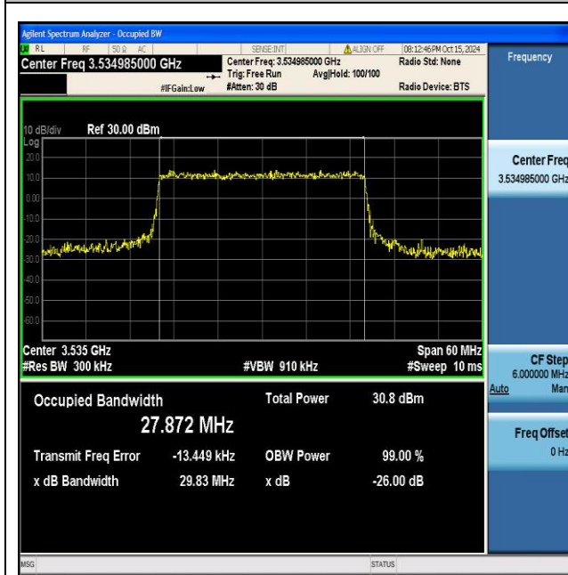
NTNV_N77-3450-3550_PC2_30_30_H_TID7_Ant1#1
