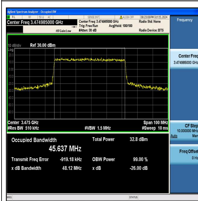
NTNV_N77-3450-3550_PC2_30_50_L_TID3_Ant1#1
