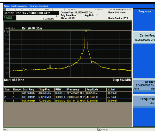
Band71-10MHz-QPSK-133422-1RB#49-PASS
