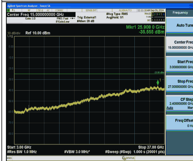
Band41-20MHz-QPSK-41490-1RB#0-3000~27000-PASS
