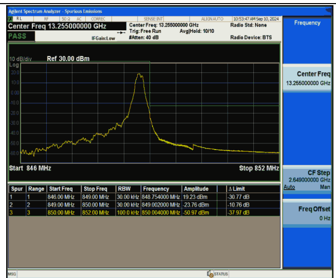
Band26(824-849)-3MHz-QPSK-27025-1RB#14-PASS
