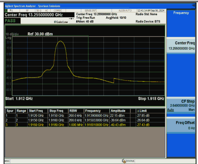
Band25-20MHz-QPSK-26590-1RB#99-PASS
