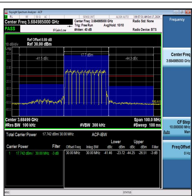
NTNV_N48_PC3_30_30_H_TID1_#1_+30_30
