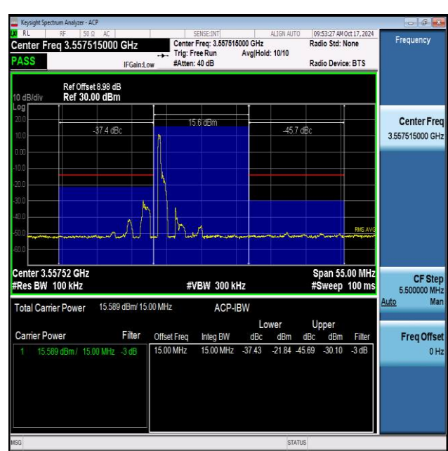
NTNV_N48_PC3_30_15_L_TID2_#1_+15_15
