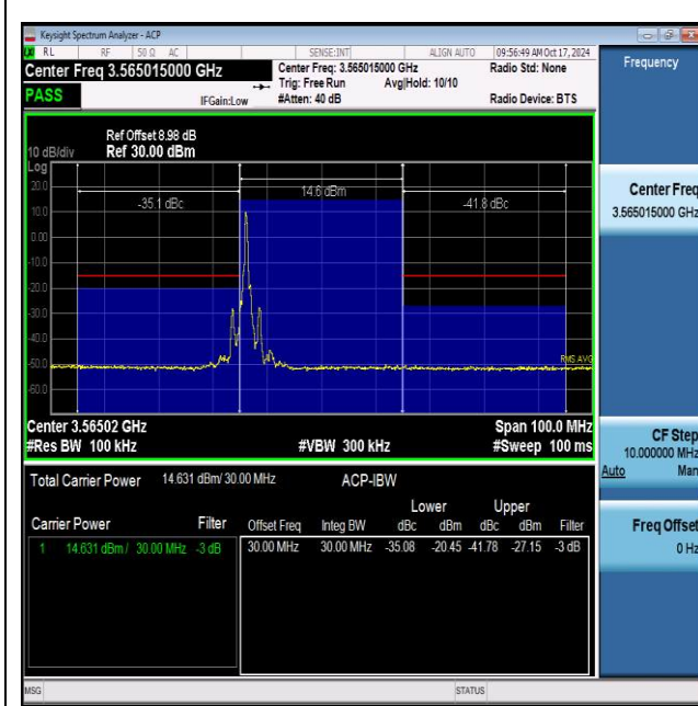
NTNV_N48_PC3_30_30_L_TID2_#1_-30_30
