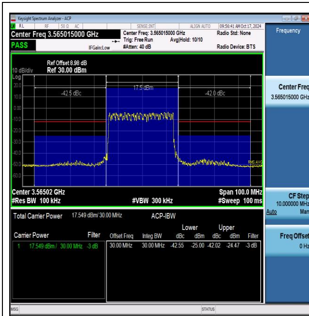
NTNV_N48_PC3_30_30_L_TID1_#1_-30_30
