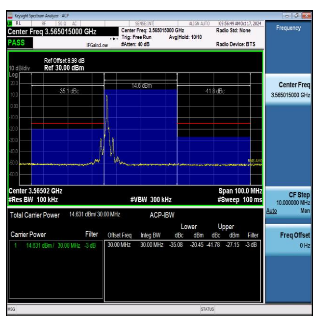
NTNV_N48_PC3_30_30_L_TID2_#1_+30_30
