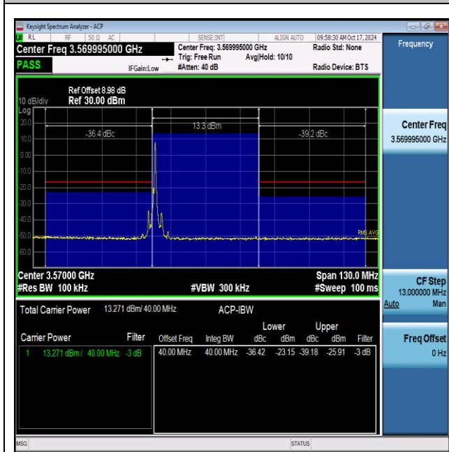
NTNV_N48_PC3_30_40_L_TID2_#1_-40_40
