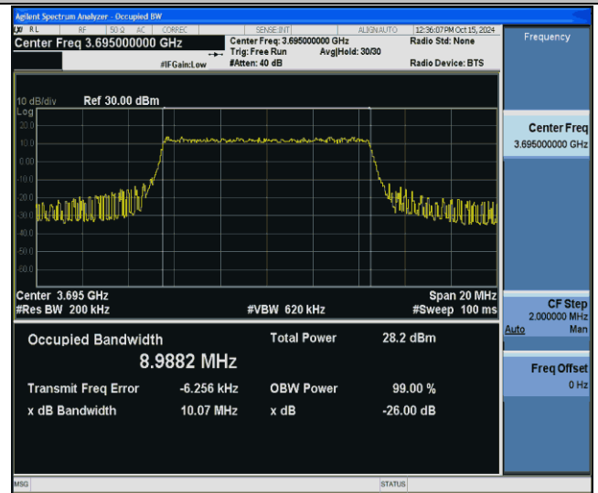
43(3600-3700)-10MHz-256QAM-44540-50RB#0-PASS
