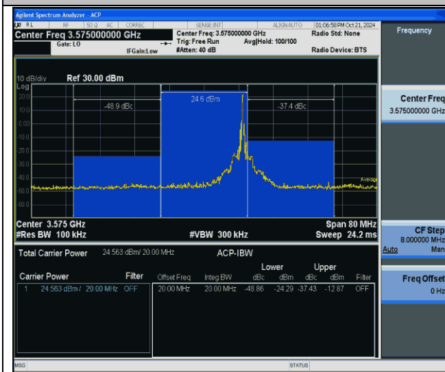
42(3550-3600)-20MHz-QPSK-43340-1RB#99-PASS
