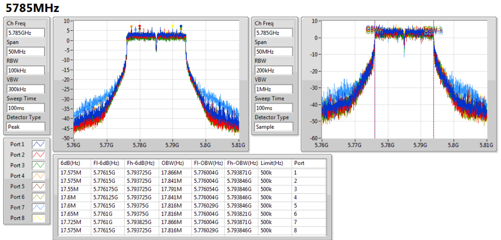
802.11ac VHT20-BF_Nss1,(MCS0)_8TX
