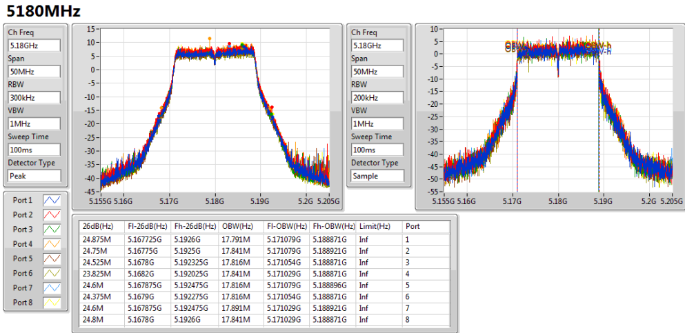
802.11ac VHT20-BF_Nss1,(MCS0)_8TX
