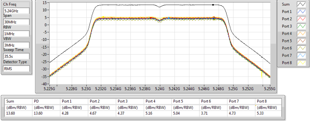
802.11ac VHT20-BF_Nss1,(MCS0)_8TX
