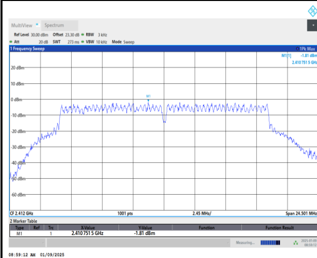
MIMO Ant 6
