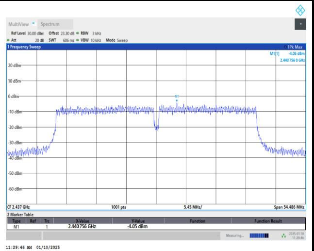
MIMO Ant 5
