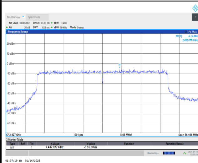
MIMO Ant 6
