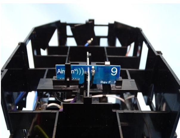
Fig.9 Antenna #9 (ZIGBEE)
