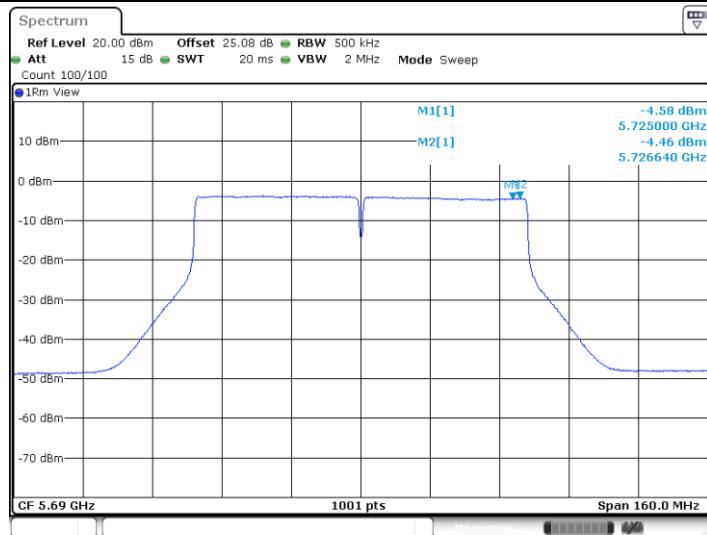
11AC80MIMO_Ant2_5690_UNII-3
