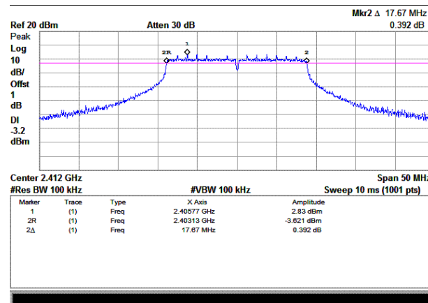
(Plot A: Channel 1: 2412MHz)
