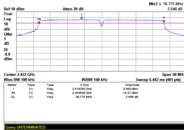
(Plot A: Channel 3: 2422MHz)
