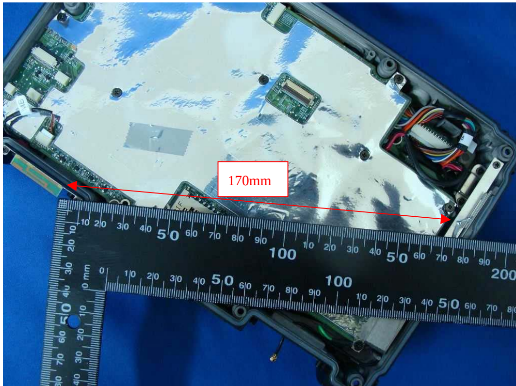
(59) EUT Photo
