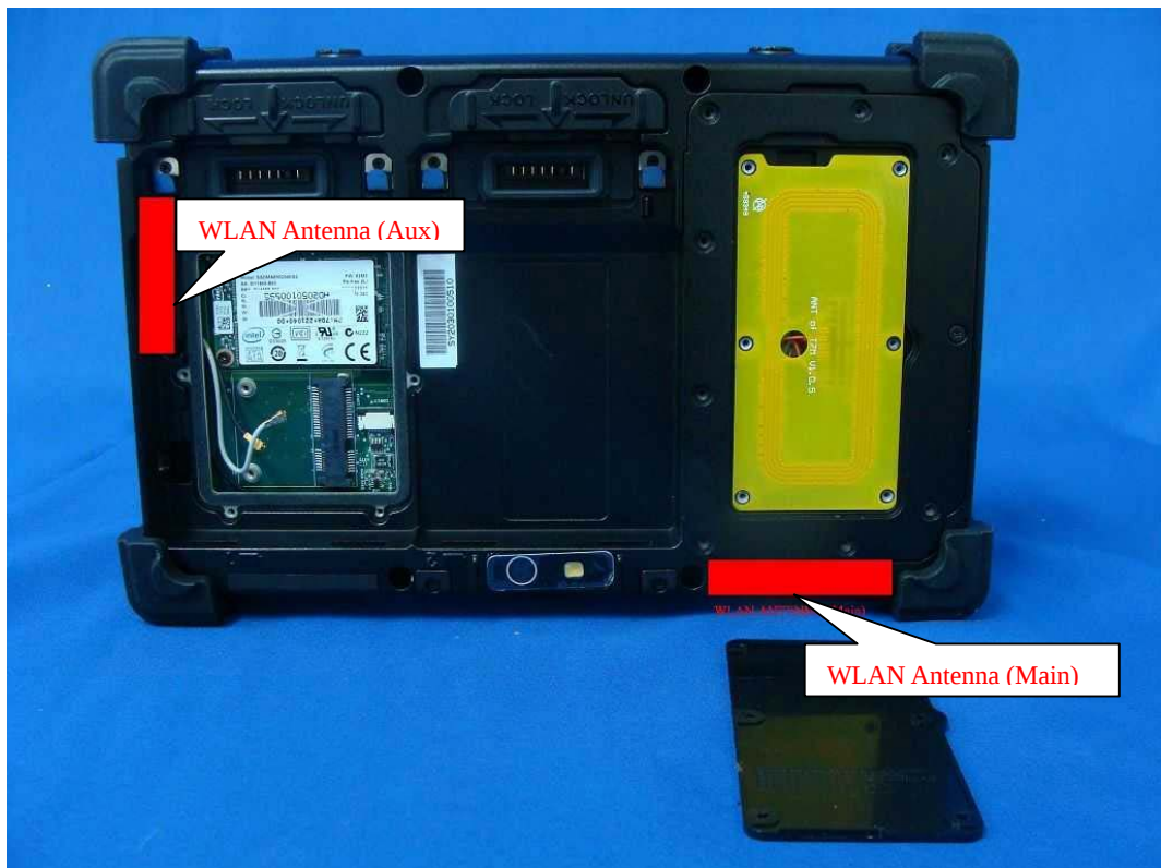
(60) EUT Photo
