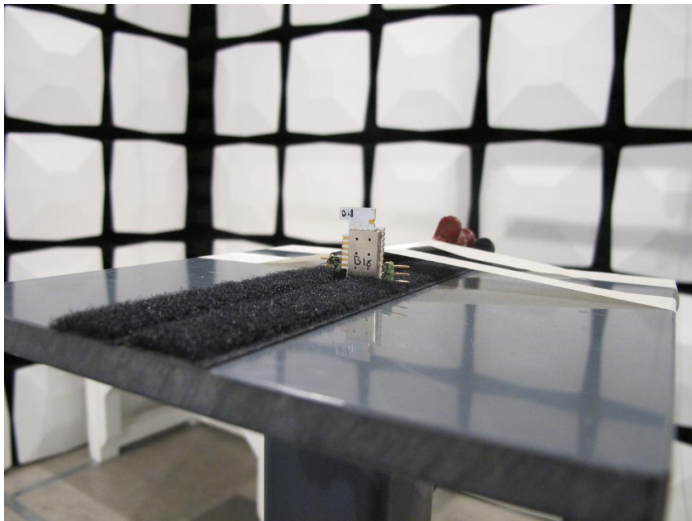
EUT in position Y
