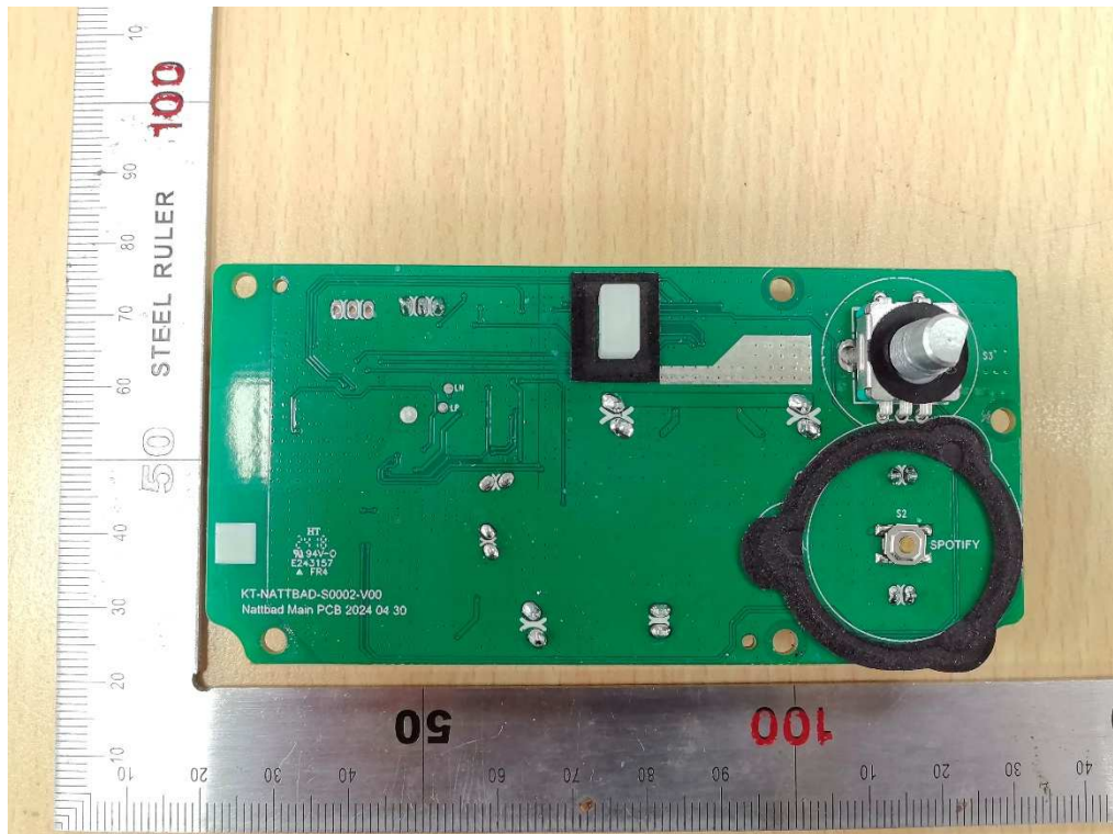
Bild / Picture 4: Mainboard view
