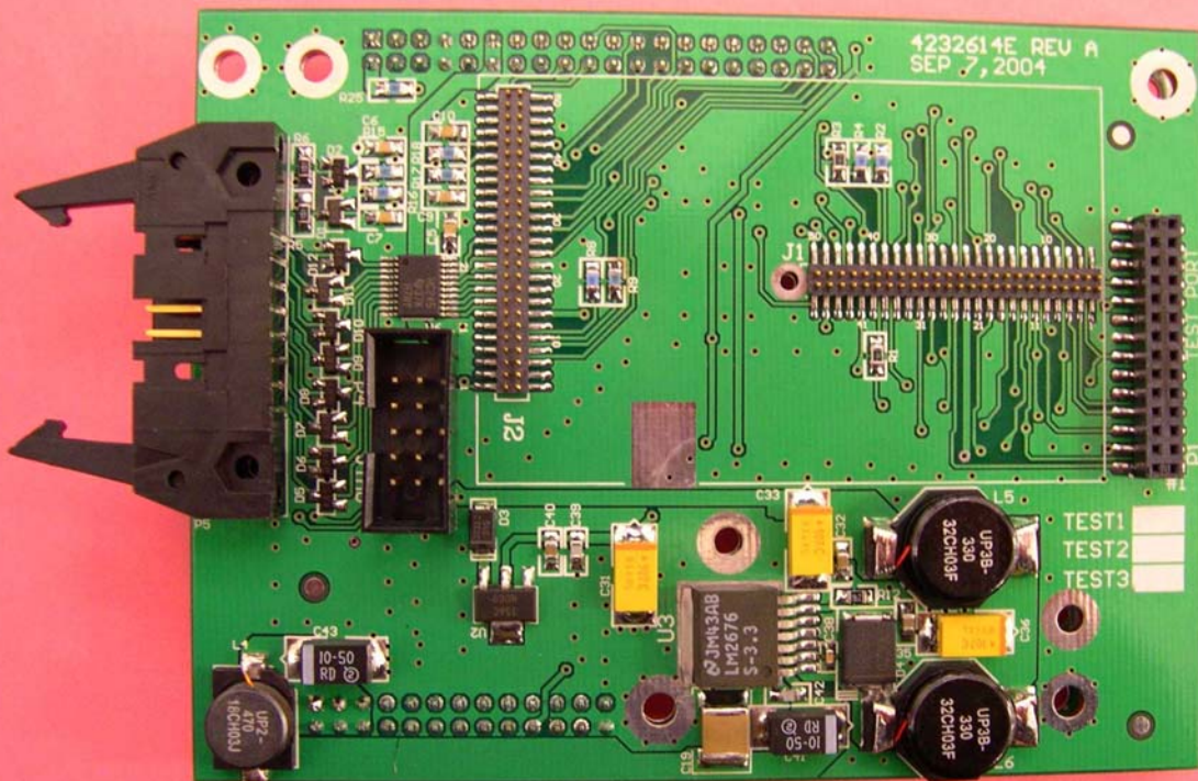
Linear Power Amplifier PCB 4232614E-A
