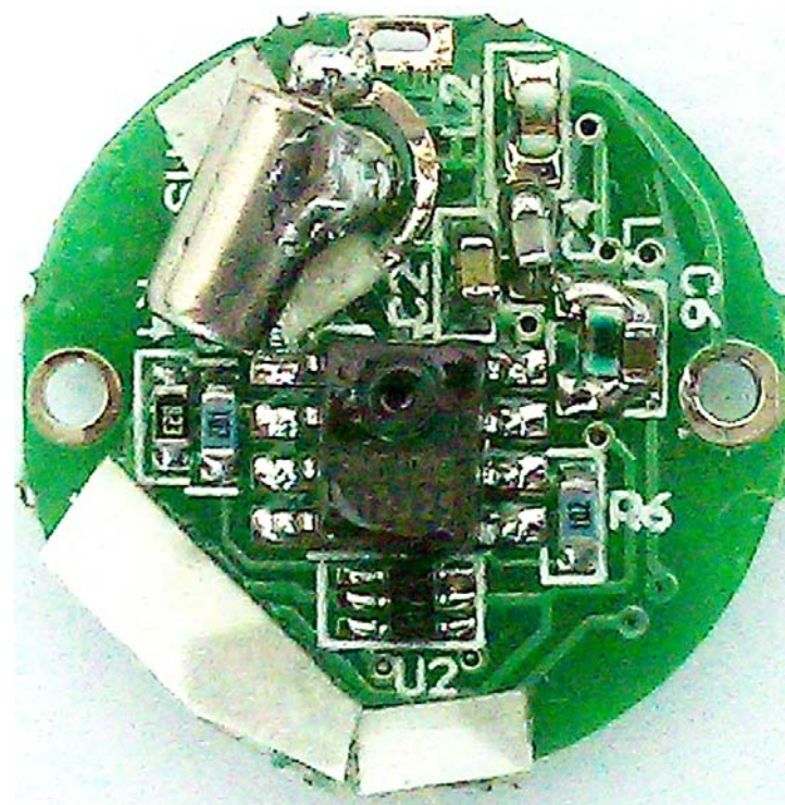
BOTTOM LAYER
