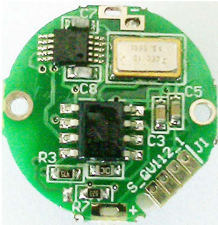
TOP LAYER
