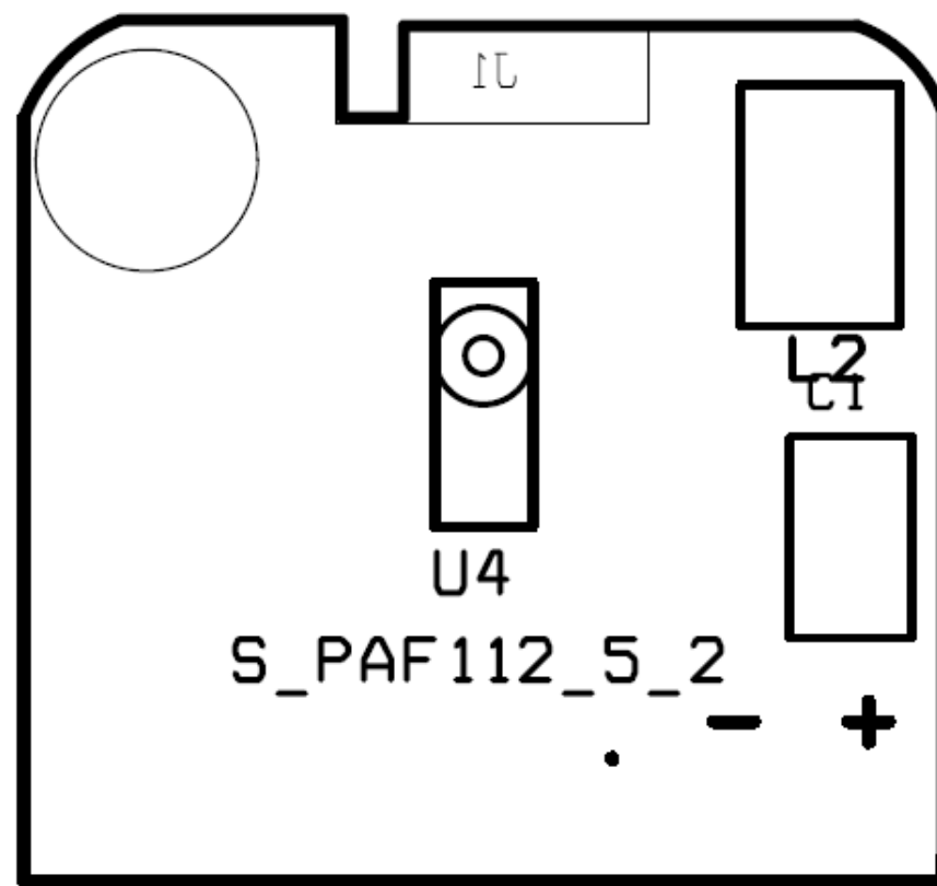
Bottom layer
