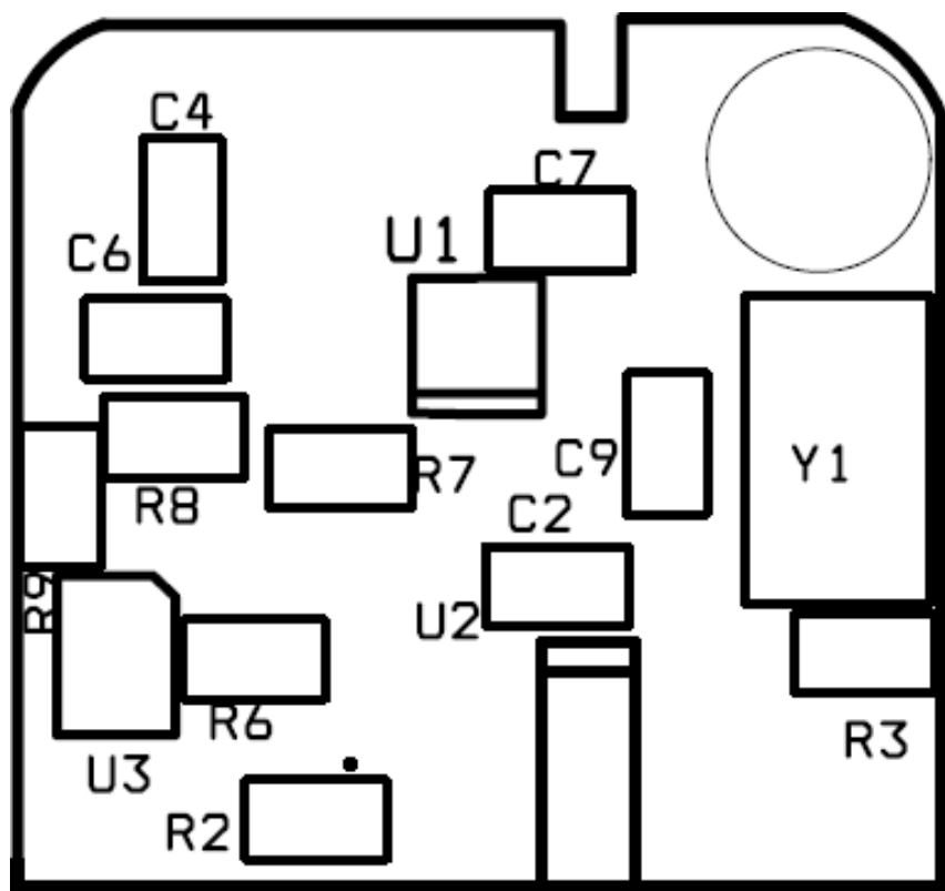
Top layer
