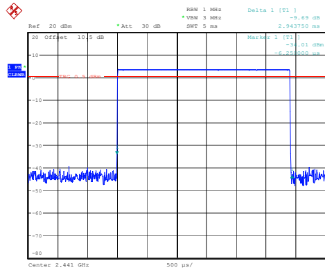
DH5_Hopping 2.944ms
