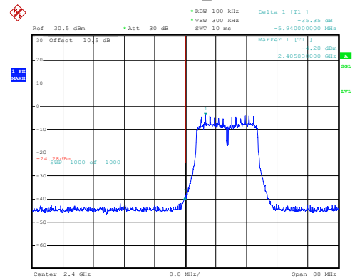
802.11n20_2412MHz
