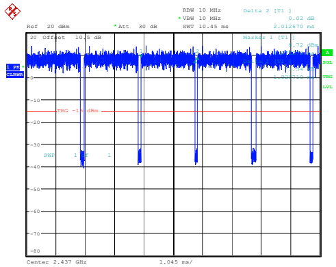
802.11n20_2437MHz
