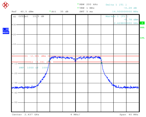
802.11g_2437MHz
