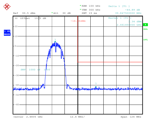
802.11b_2462MHz
