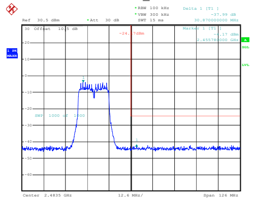
802.11n20_2462MHz
