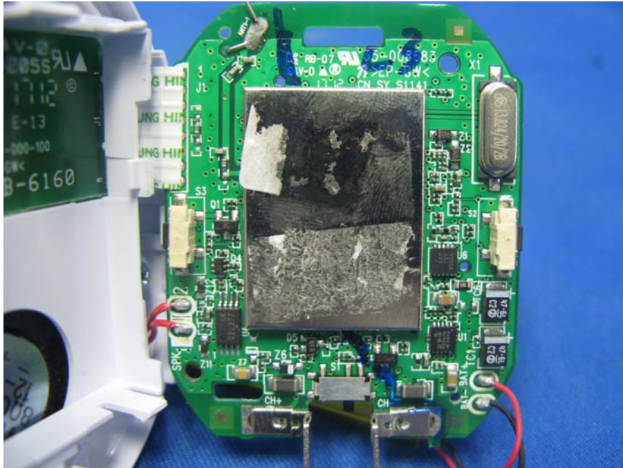
Pendant Main PCB comp side
