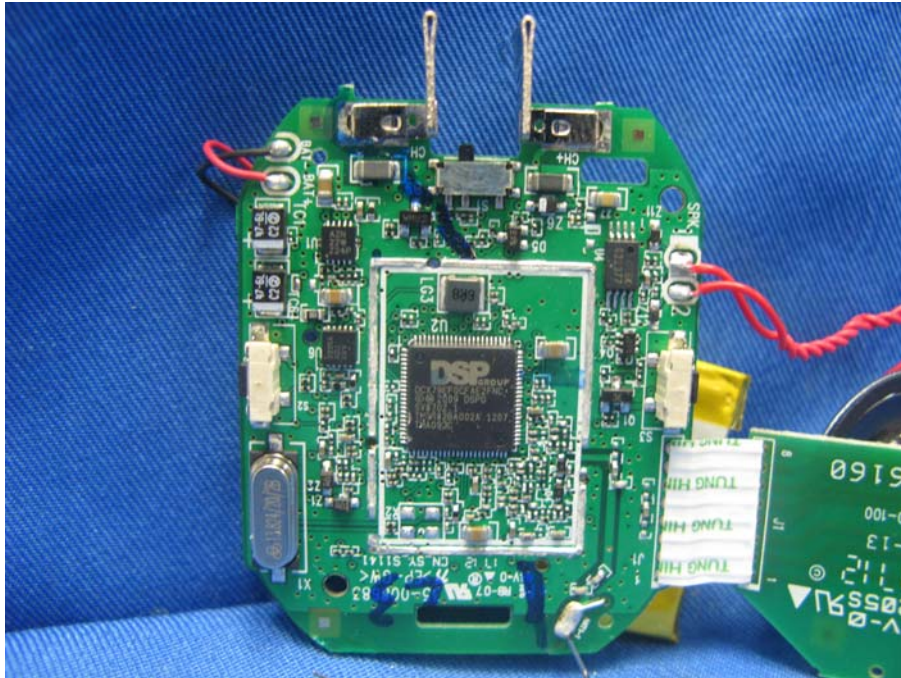
Pendant Oscillator PCB comp side
