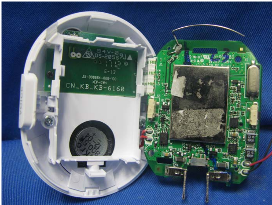
Pendant assembly (View 2)
