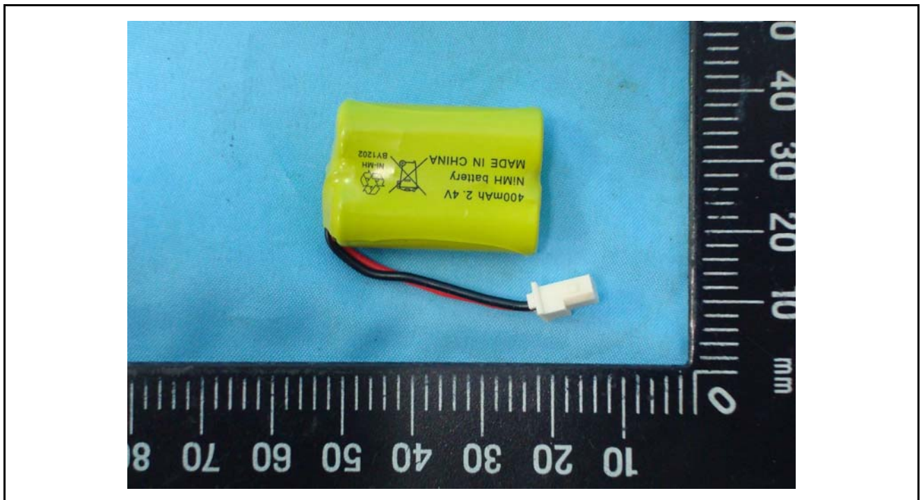
EUT Photo ( 4 )
