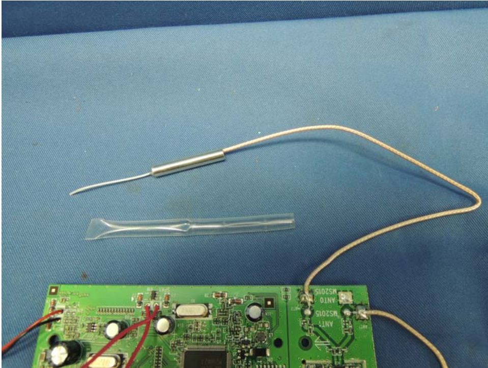
Deskset Antenna 1
