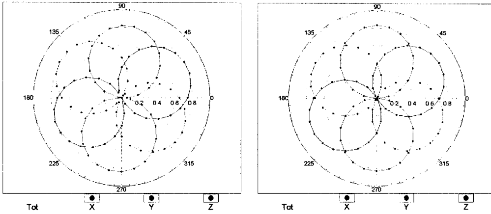
f=1800 MHz,R22
