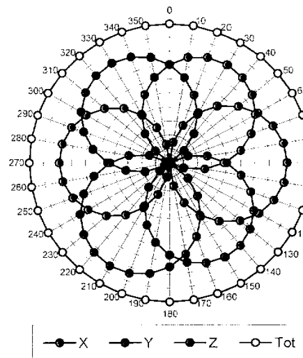
f = 600 \text{ MHz} , TEM ifi110EXX
