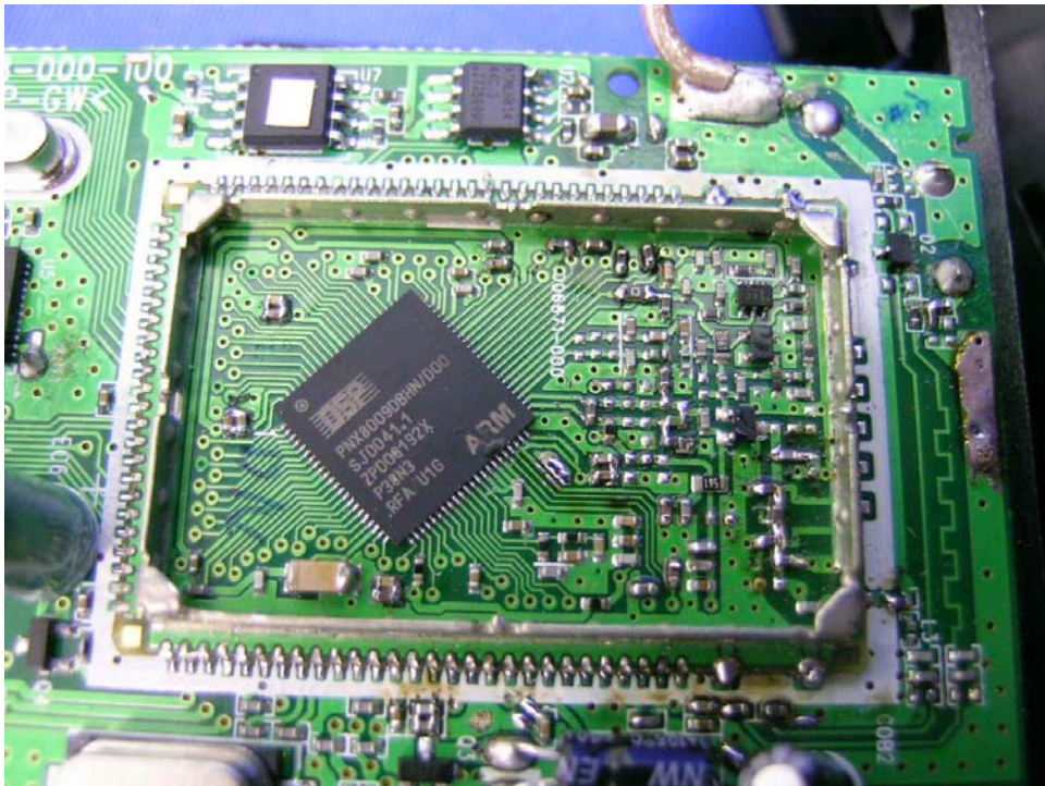
Base Unit 1.9GHz RF Module
