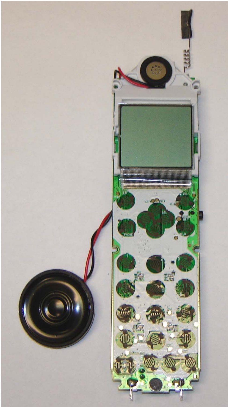
AT&T E5804 - Handset PCB
