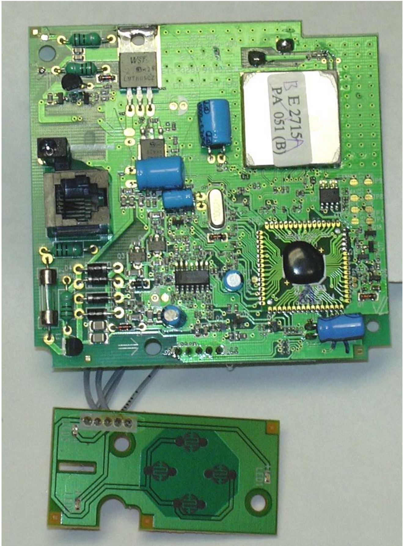
AT&T E2715B Base PCB
