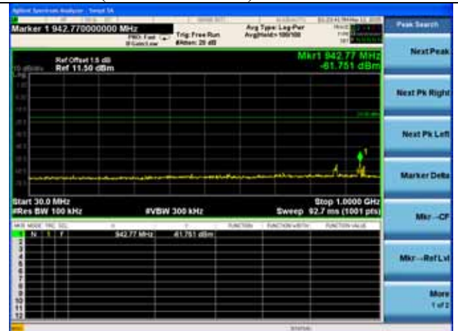
2402MHz(30MHz – 1GHz)
