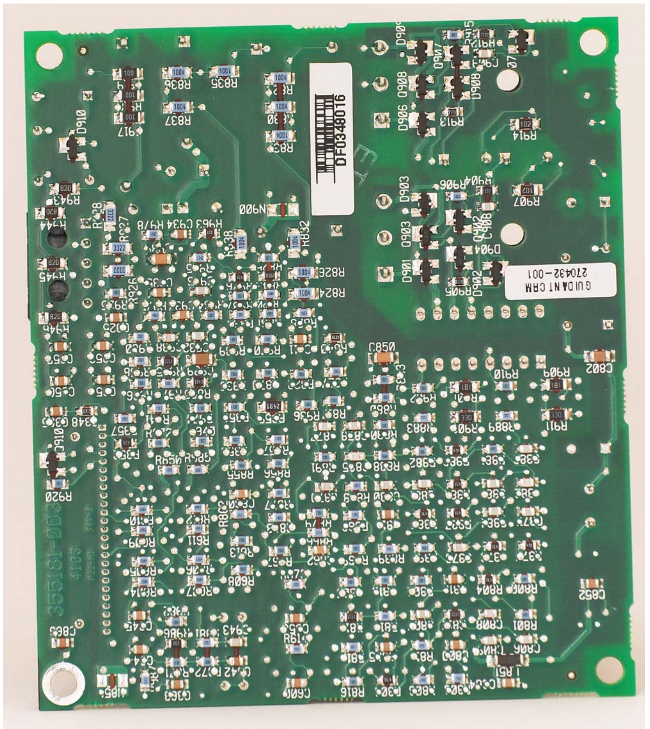
3120 Zoom Latitude Programming System Inductive Module Bottom Side
