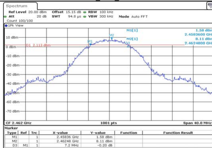
11B_Ant1_2462
