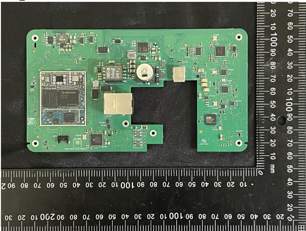
(14) EUT Photo_M202404002
