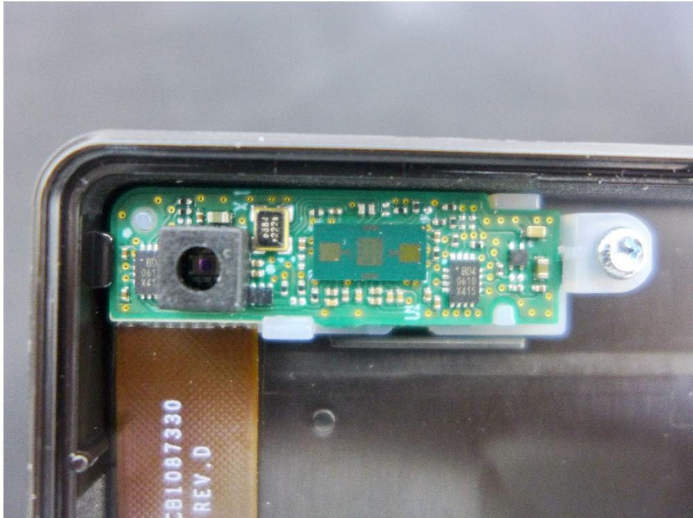
(7) EUT Photo_M202404002
