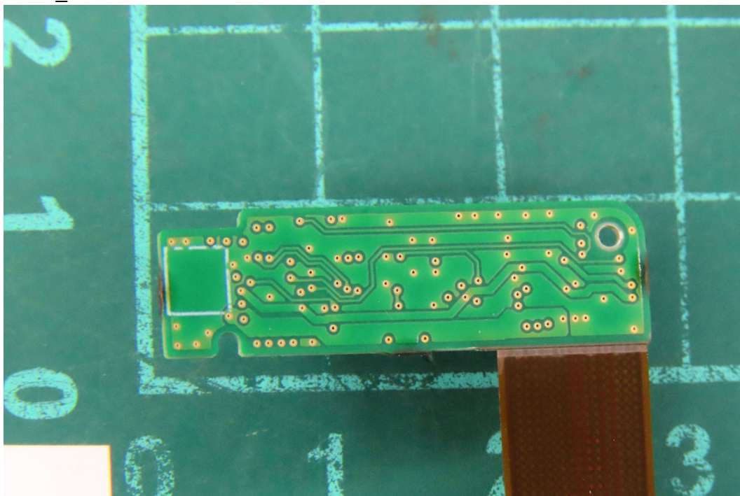
(9) EUT Photo_M202404002
