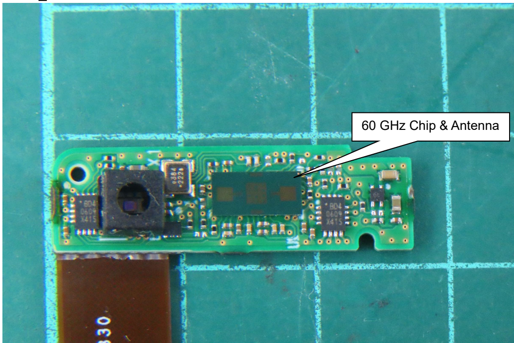
(8) EUT Photo_M202404002
