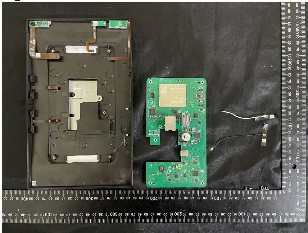
(6) EUT Photo_M202404002
