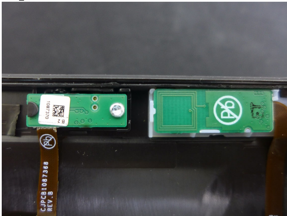
(10) EUT Photo_M202404002
