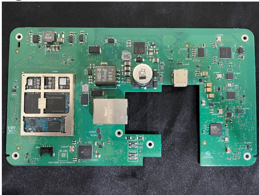
(16) EUT Photo_M202404002
