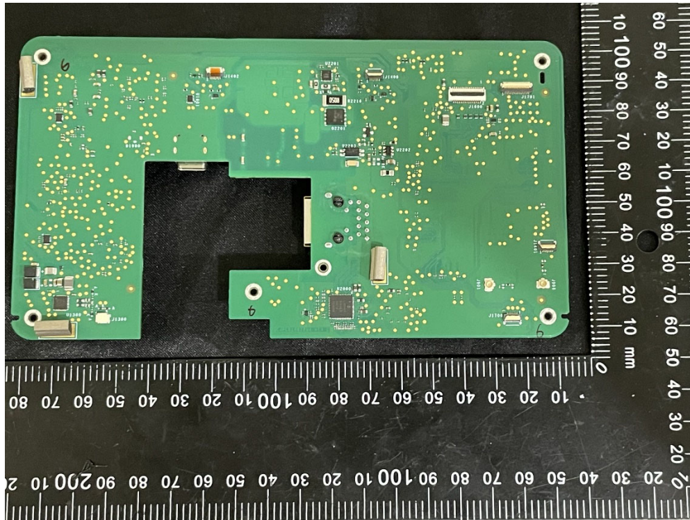
(15) EUT Photo_M202404002
