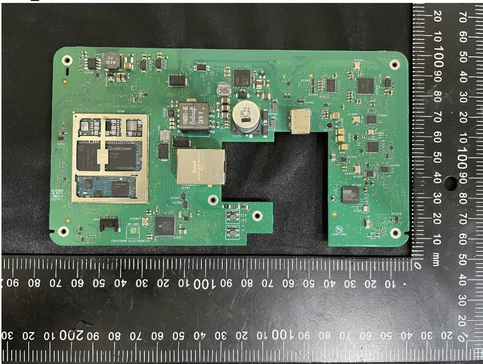
(12) EUT Photo_M202404002
