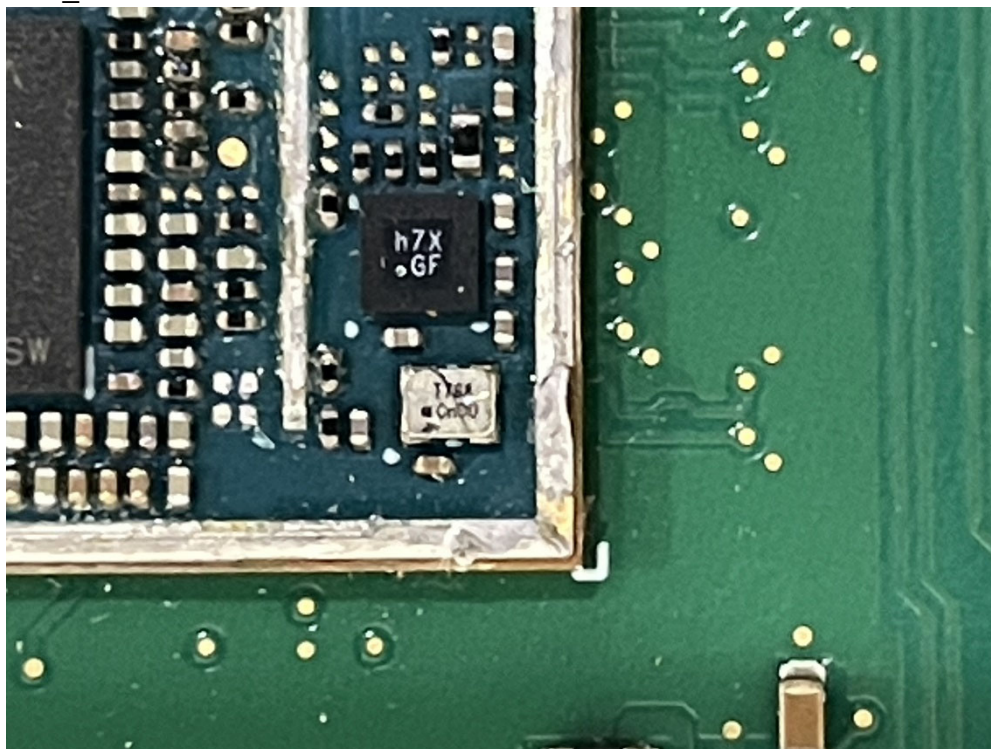
(19) EUT Photo_M202404002
