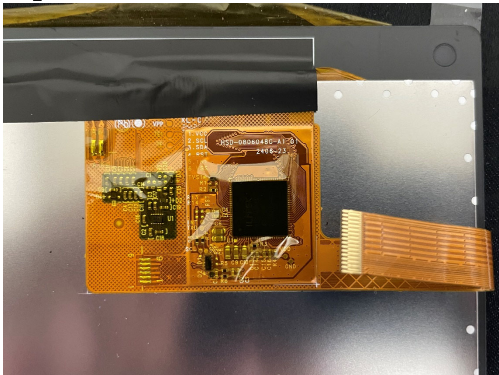
(24) EUT Photo_M202404001
