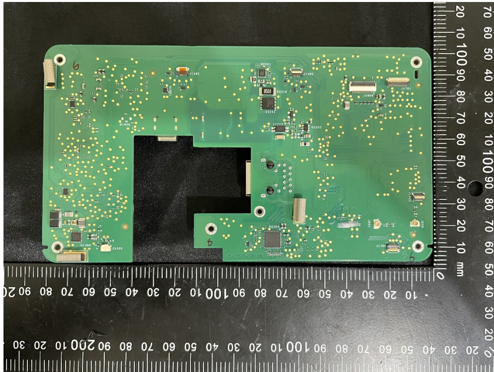
(13) EUT Photo_M202404002
