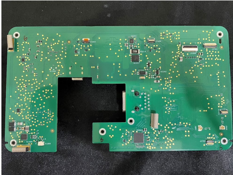
(17) EUT Photo_M202404002
