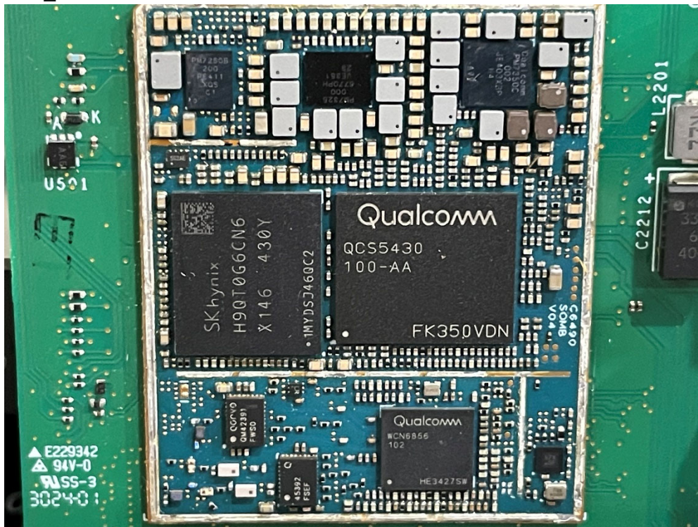
(18) EUT Photo_M202404002
