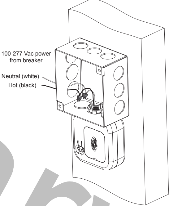
ZUMMESH-JBOX-PSU Wiring
