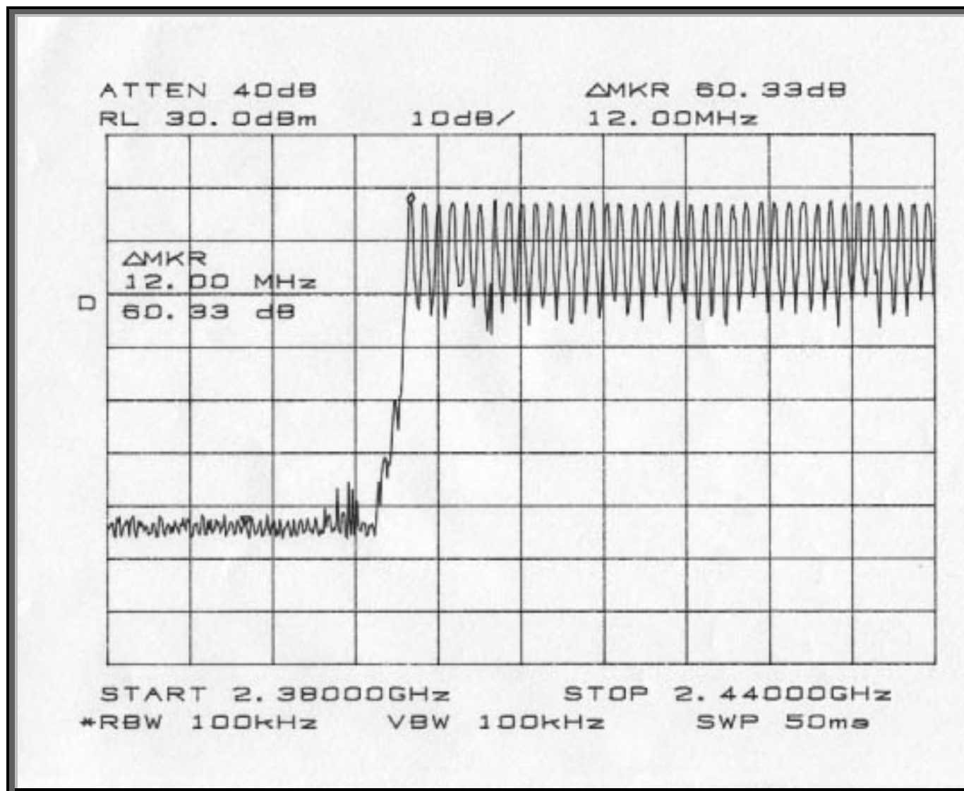
Lower Band Edge
