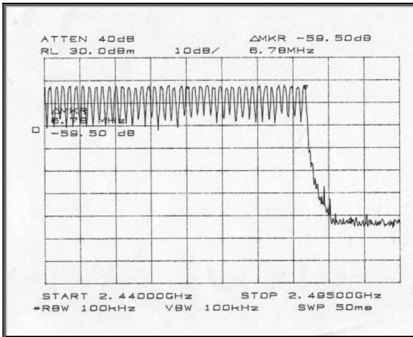
Upper Band Edge
