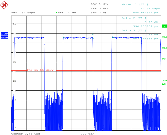
Figure 8.6-1: Pulse width for BLE
