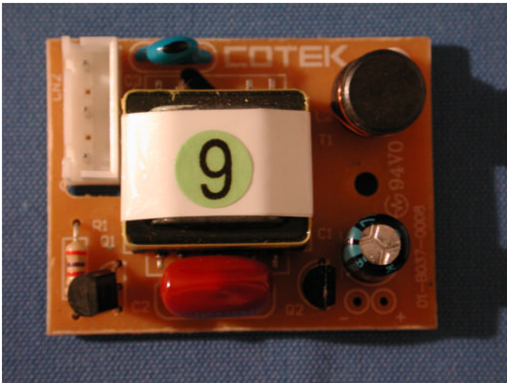
(16) EUT Photo
