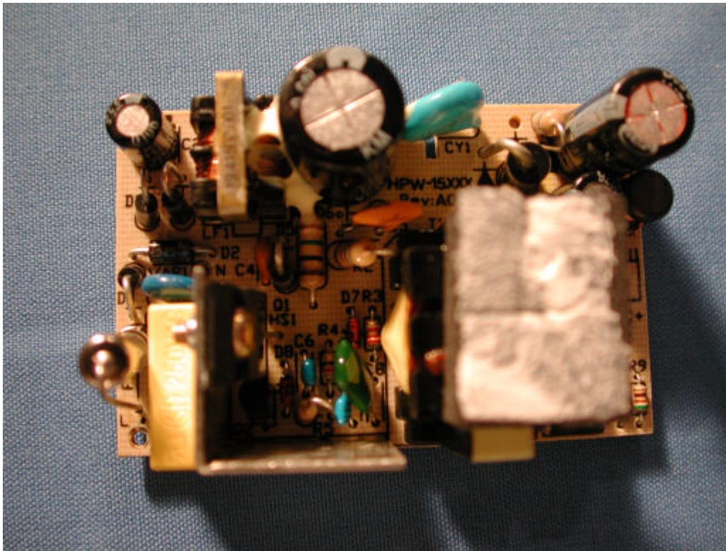
(24) EUT Photo
