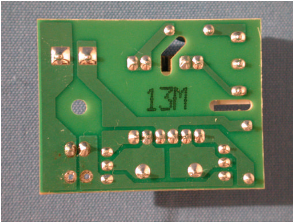
(18) EUT Photo
