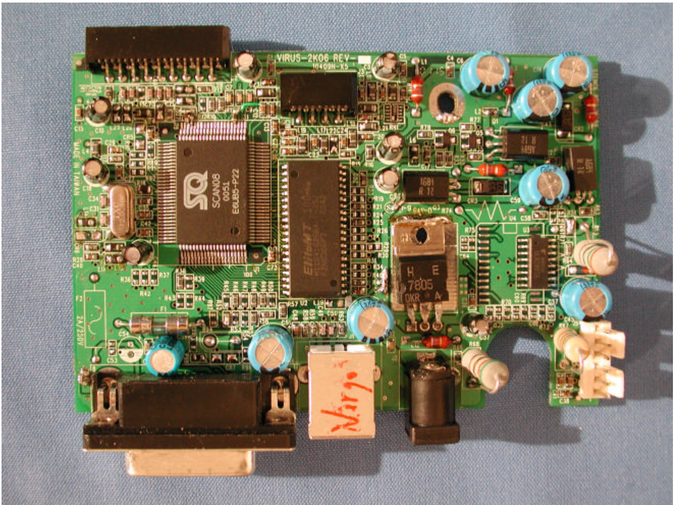
(19) EUT Photo
