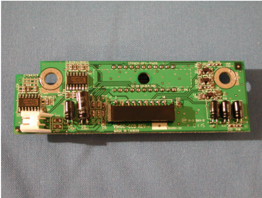
(14) EUT Photo
