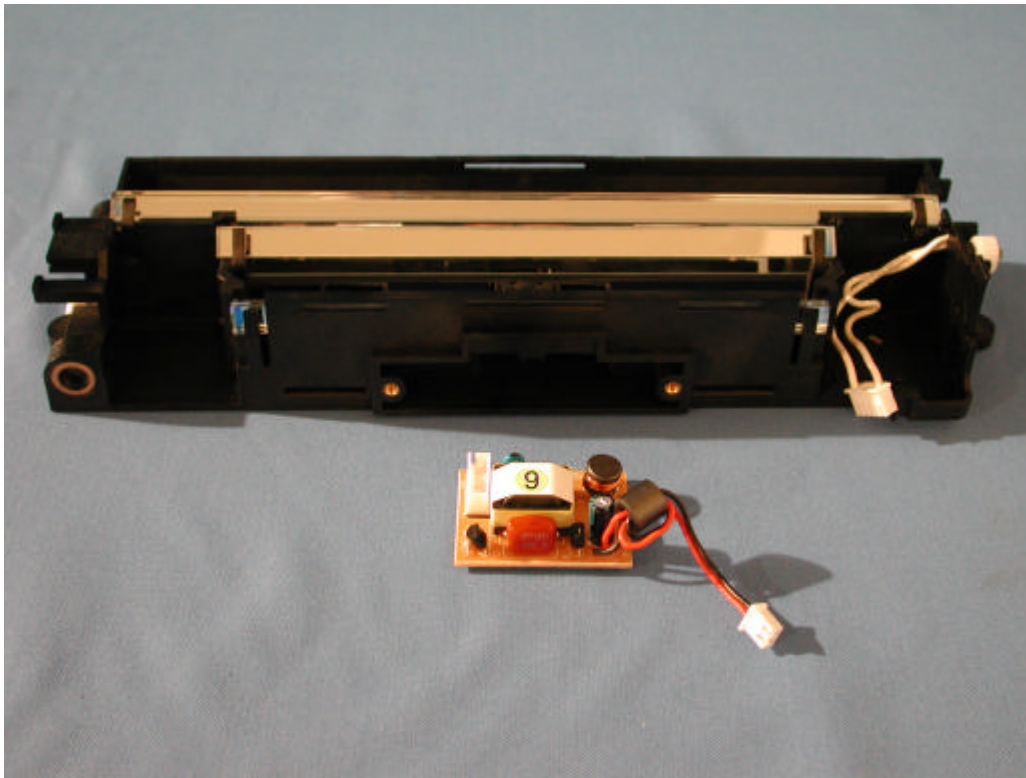
(16) EUT Photo
