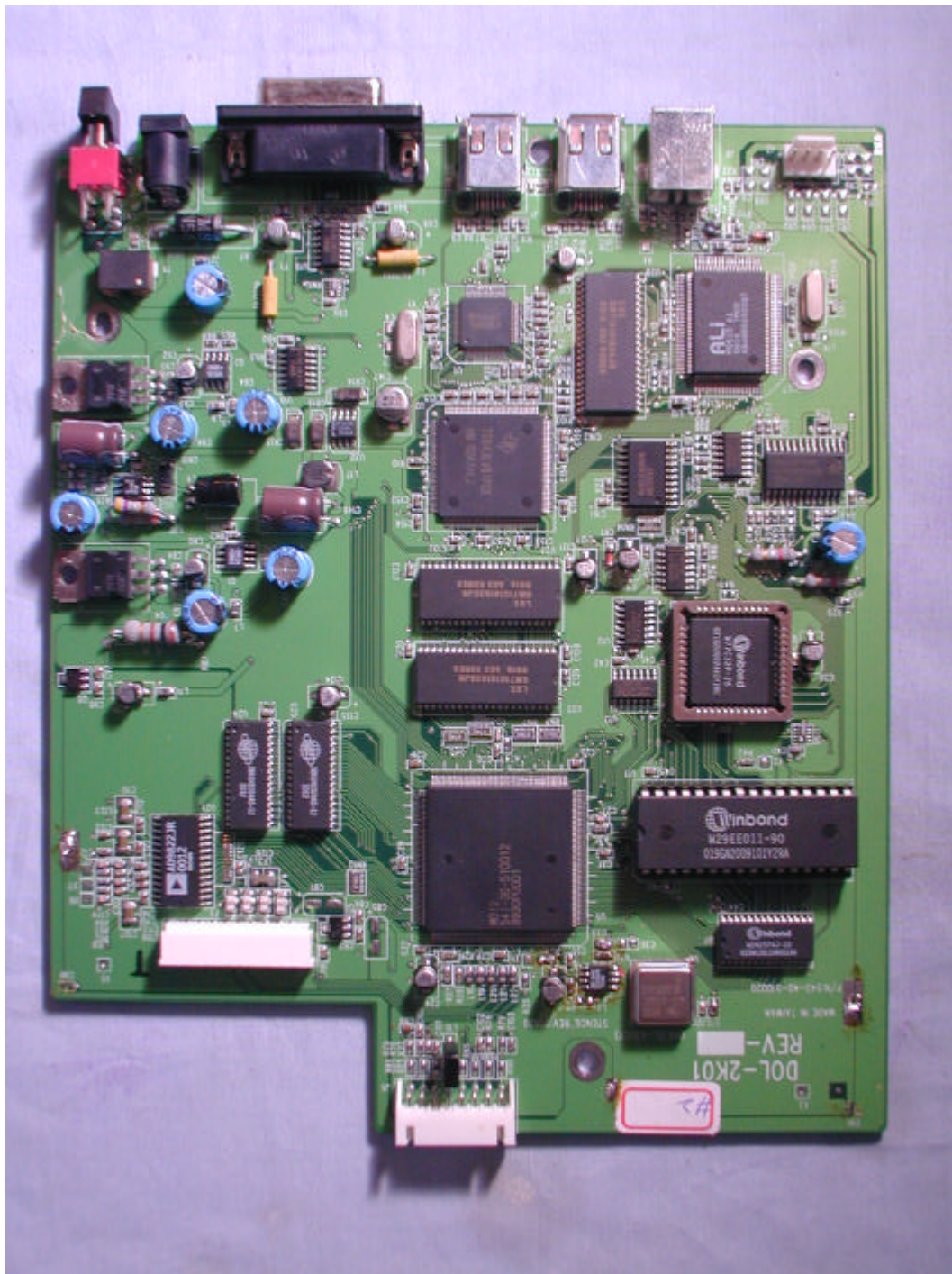
(18) EUT Photo
