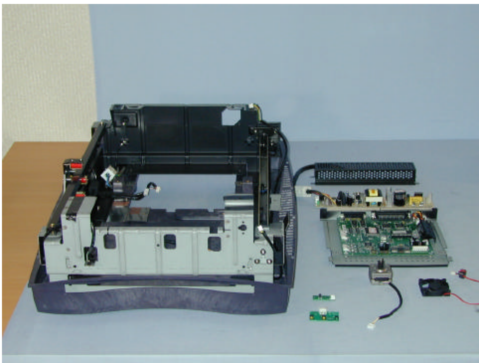
(6) EUT Photo
