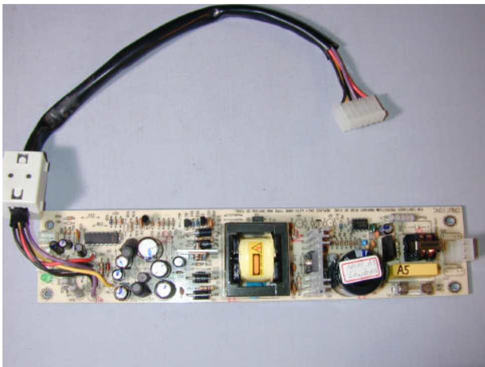
(14) EUT Photo
