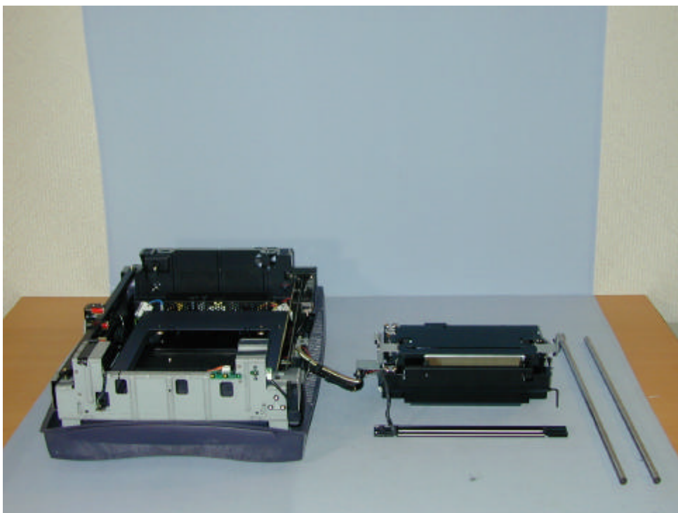
(4) EUT Photo
