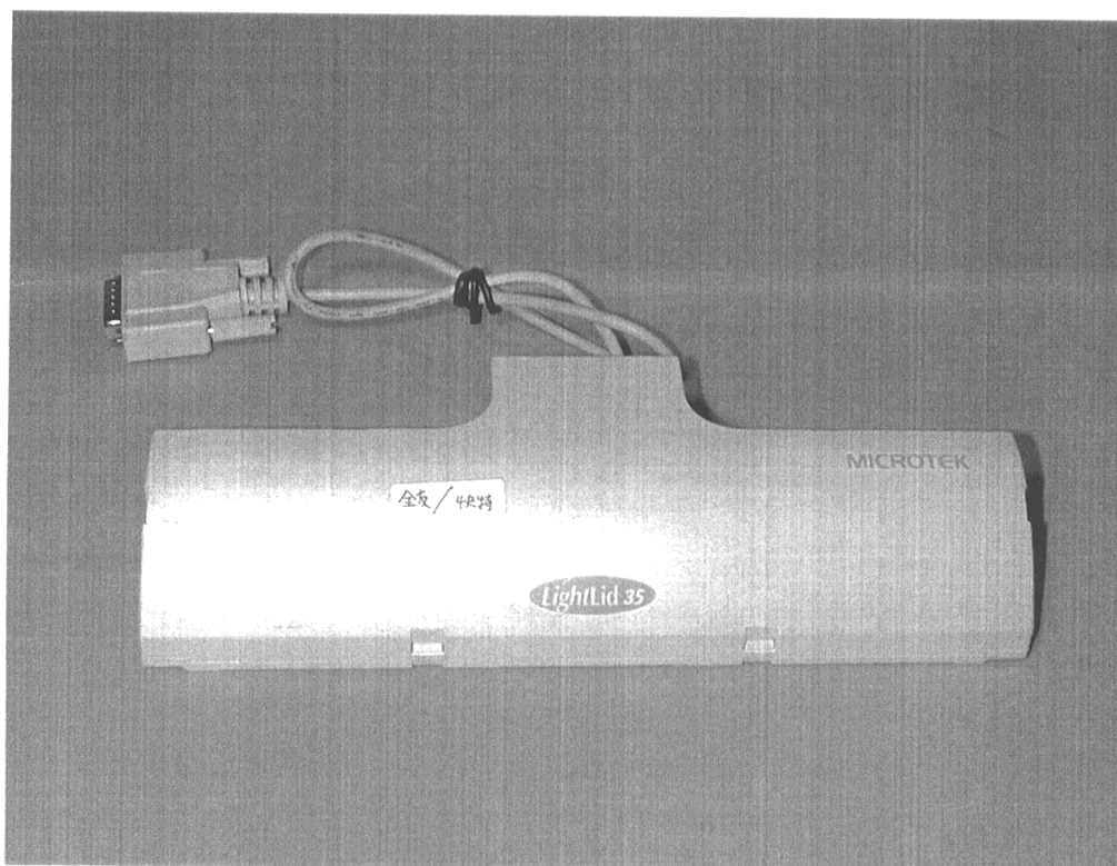
(30)EUT Photo(Mode 1: Li Shin & Mode 2: Bestec)
