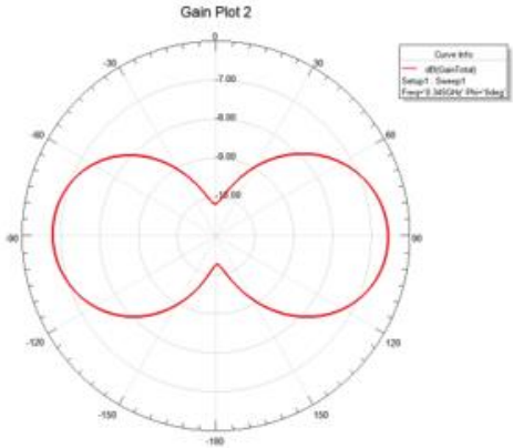
345 · 000MHz E1
