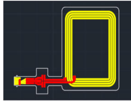
NFC Antenna Layout
