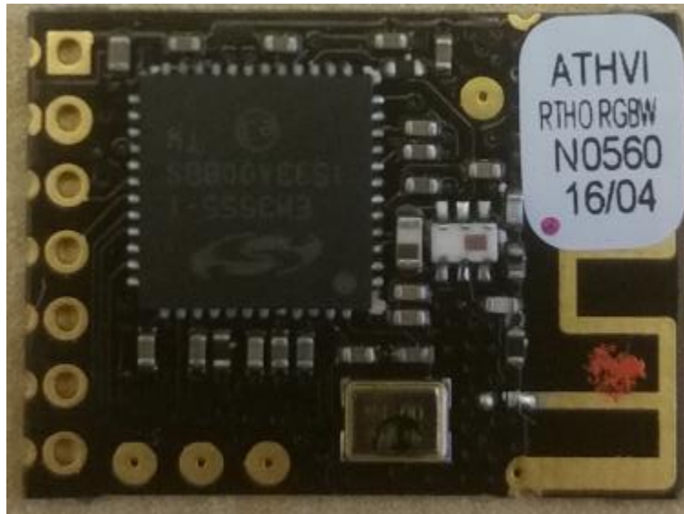
Aether module photo
